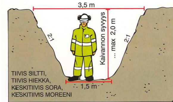
Esimerkkikuva hyväksytystä kaivannosta yleisillä maalajeilla. pehmeää
