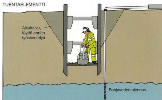
Esimerkkikuva hyväksytystä tuentaelementeillä perustetusta kaivannosta.
