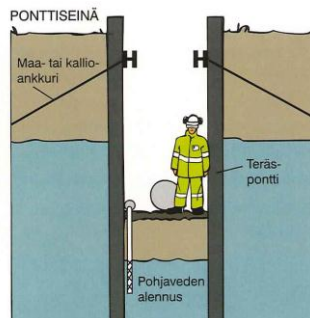
Esimerkkikuva hyväksytystä ponttiseinällä tuetusta kaivannosta
