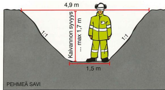
Esimerkkikuva hyväksytystä kaivannosta maaperän ollessa savea.
